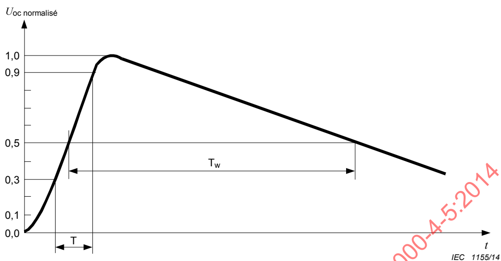
Figure A.2 – Forme d'onde de tension en circuit ouvert (10/700 \mu\text{s} )
