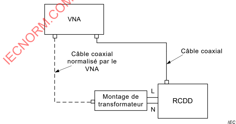
Figure 10 – Montage pour l'évaluation de la perte d'insertion totale du système de couplage d'injection
