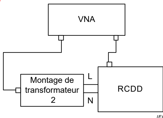
Figure 8b) – Montage de mesure de la perte d'insertion pour la mesure A_{13} sur le montage de transformateur
