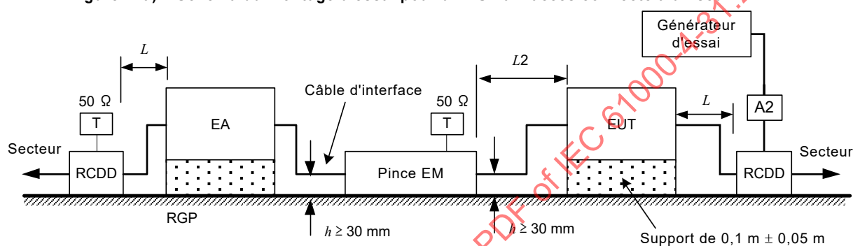
Figure 14a) – Schéma du montage d'essai pour un EUT à 2 accès connecté à un seul RCDD
