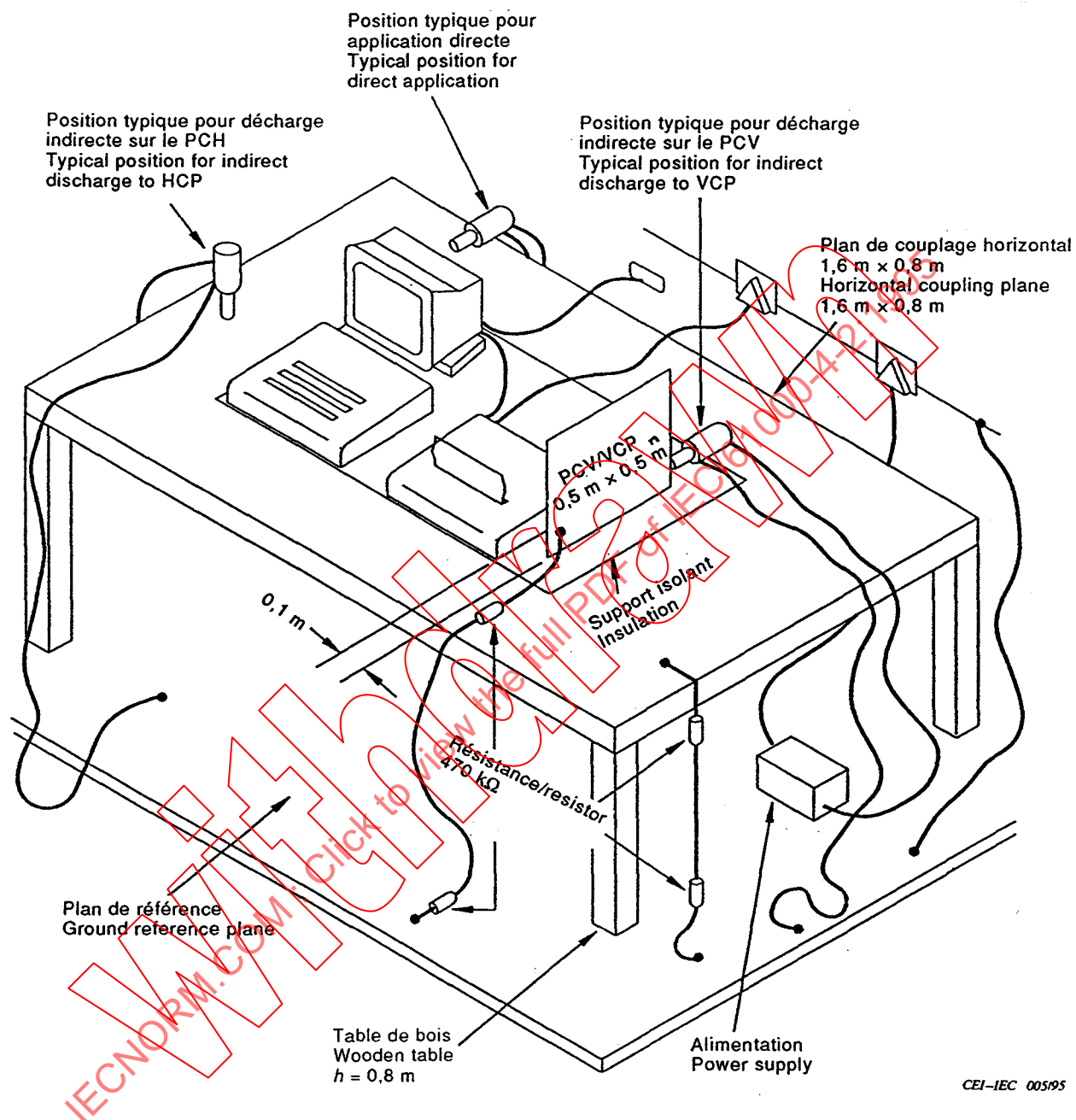
Figure 5 – Exemple d'installation d'essai pour matériel de table, essais en laboratoire Example of test set-up for table-top equipment, laboratory tests
