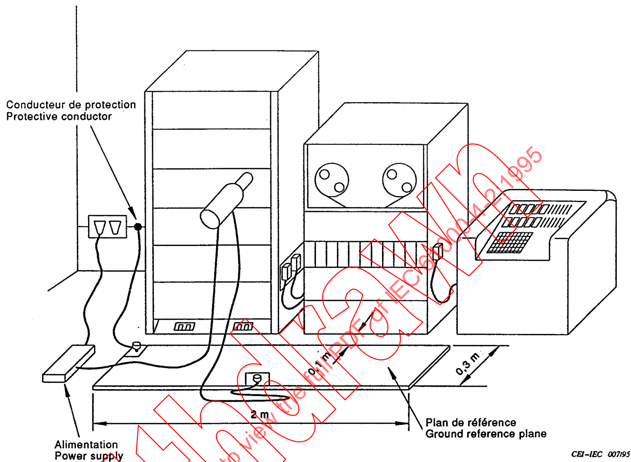
Figure 7 – Exemple d'installation d'essai pour matériels posés au sol, matériels installés Example of test set-up for floor-standing equipment, post-installation tests
