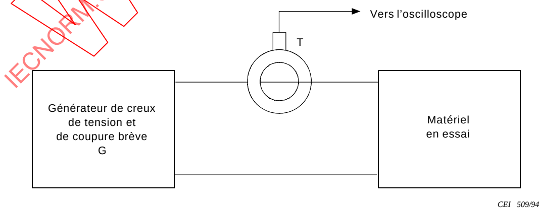
Figure A.2 - Circuit pour la détermination du courant d'appel crête d'un matériel en essai
