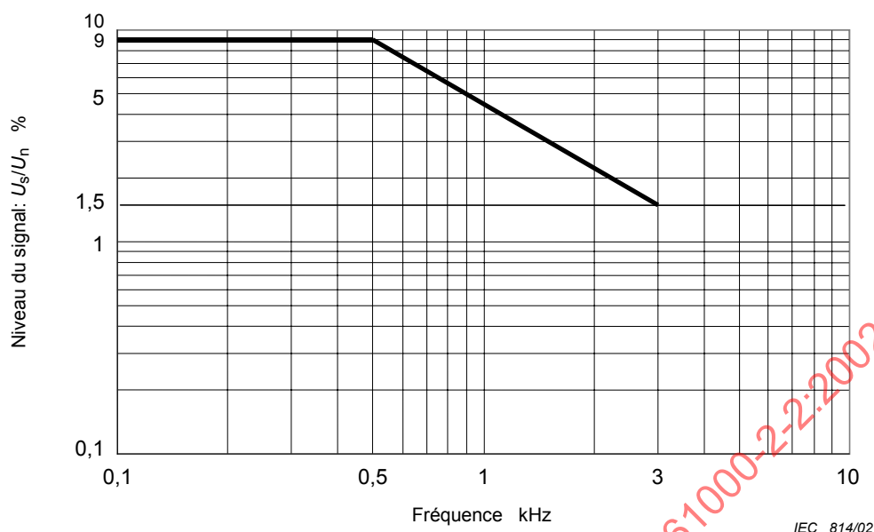
Figure 3 – Courbe «de Meister» pour les systèmes de télécommande centralisée dans les réseaux publics (100 Hz à 3 000 Hz)
