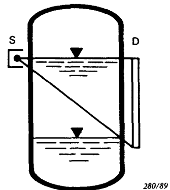
Figure 3 - Source ponctuelle et détecteur allongé
