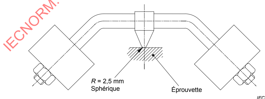
Figure 8 – Appareil pour l'essai à la bille
