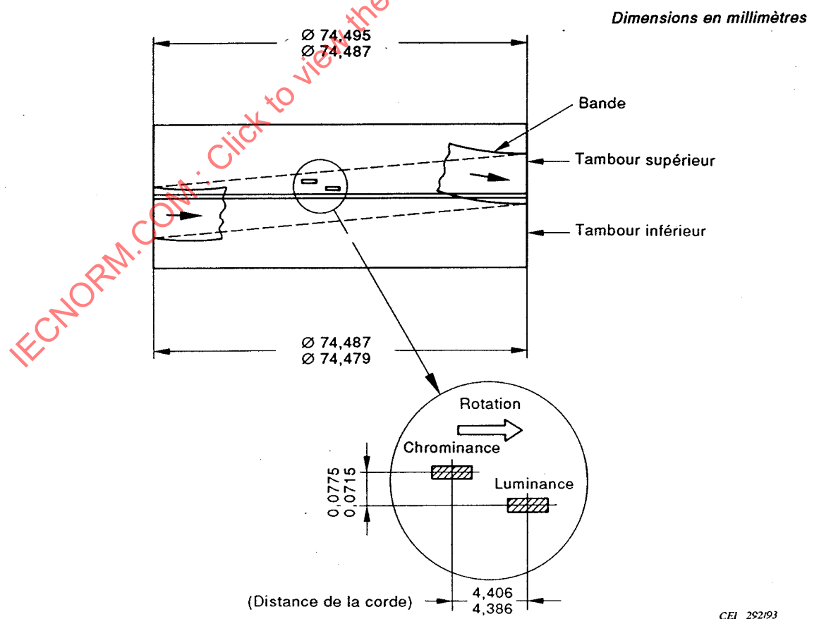
Figure 2 – Diamètres du tambour et vue de côté des pièces polaires du dispositif de balayage
