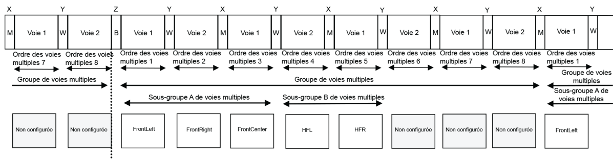
Figure 1 – Exemple: groupe et sous-groupes de voies multiples
