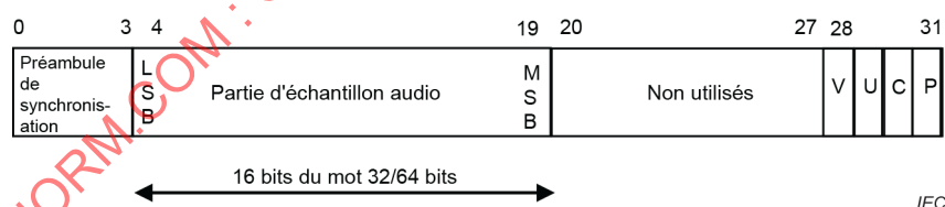
Figure 3 – Sous-trame du mode 32/64 bits
