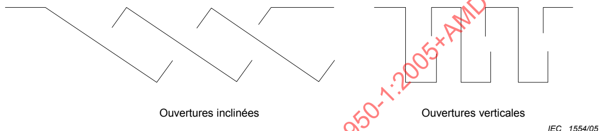
Figure 4B – Exemples de coupes d'ouvertures empêchant un accès vertical
