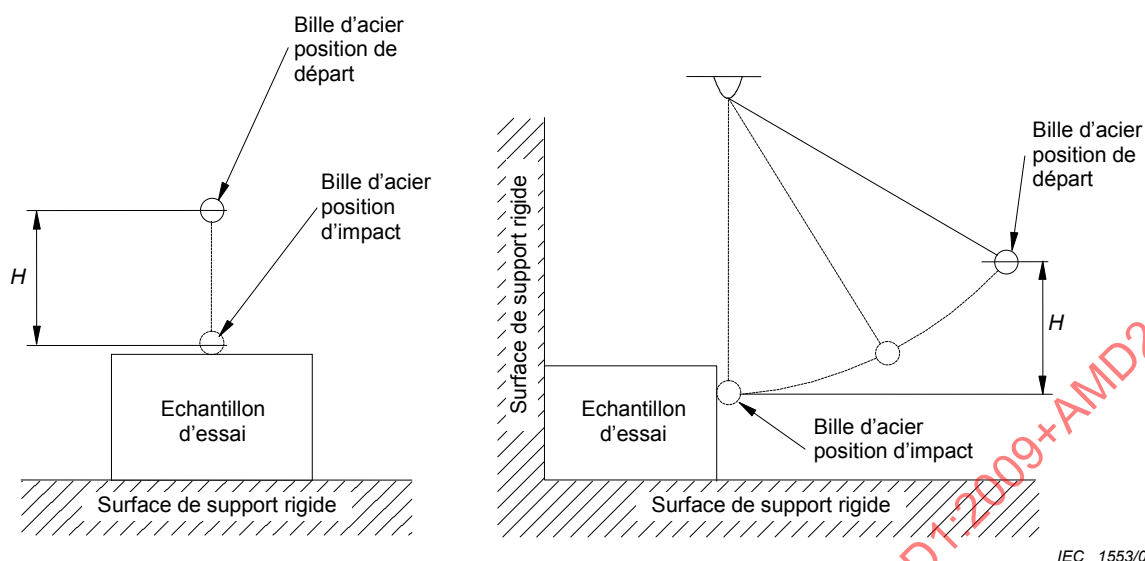
Figure 4A – Essai de choc utilisant la sphère d'acier
