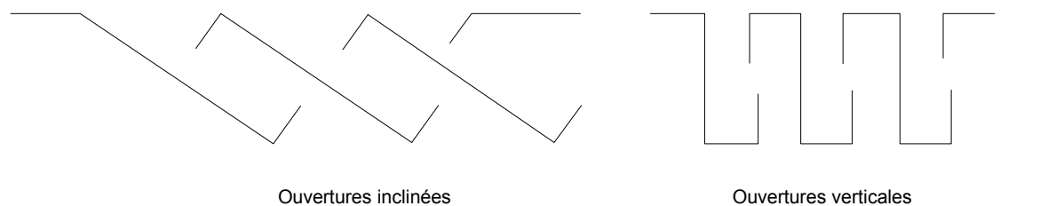
Figure 4B – Exemples de coupes d'ouvertures empêchant un accès vertical
