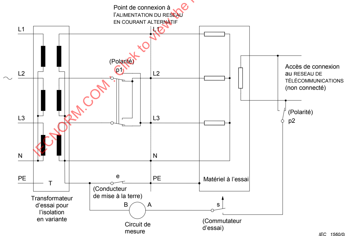
Figure 5A – Circuit d'essai pour le courant de contact d'un matériel monophasé sur des schémas d'alimentation TN étoile ou TT
