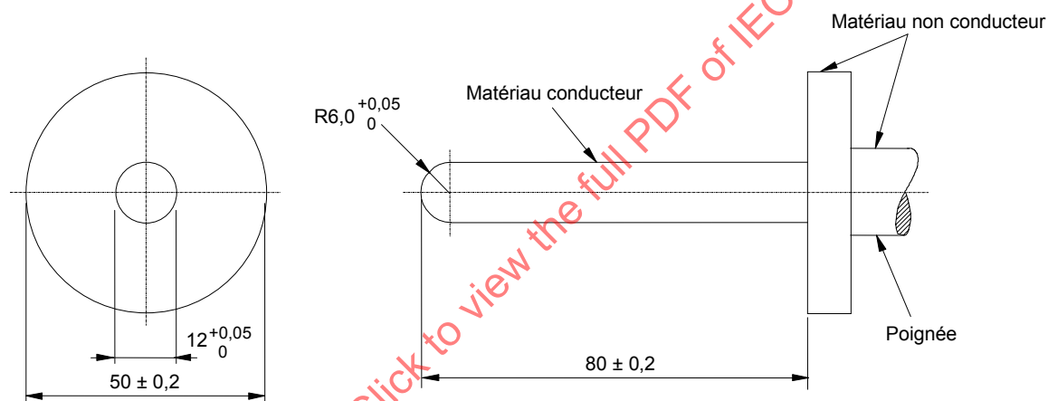
Figure 2B – Broche d'essai
