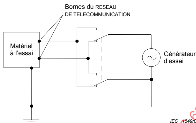
Figure 2G – Générateur d'essai
