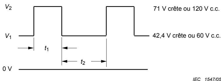
Figure 2E – Tensions dans les circuits TBTS dans les conditions de premier défaut
