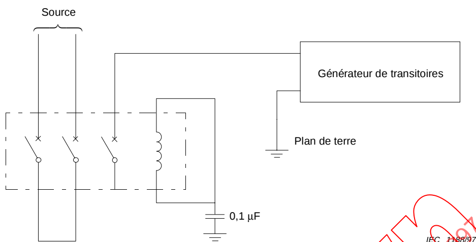
Figure 4 – Circuit d'essai pour la vérification de l'influence des transitoires dans le circuit principal (mode commun)
