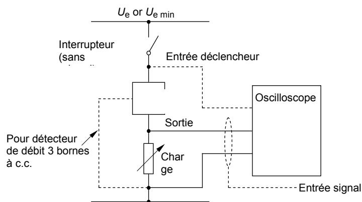
Figure 3 – Circuit d'essai pour la vérification du retard à la disponibilité
