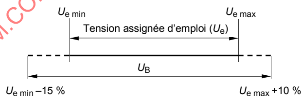
Figure 2 – Relation entre U_e et U_B
