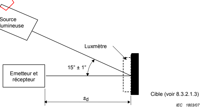
Figure 11d – Type D, émetteur-récepteur et cible
