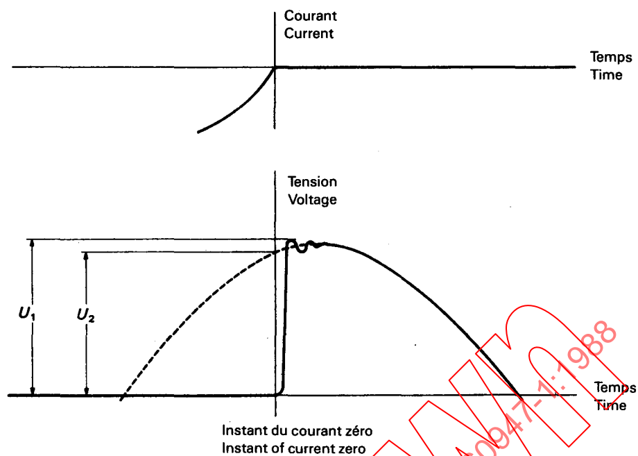
FIG. 7. — Représentation schématique de la tension de rétablissement entre les contacts de la première phase qui coupe (voir paragraphe 8.3.3.5.2 e )) dans des conditions idéales.
