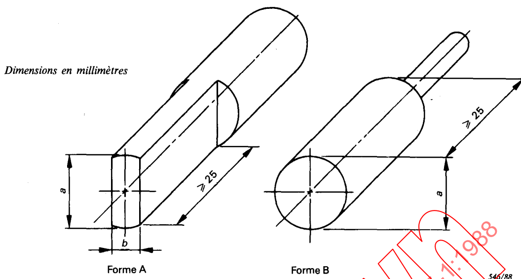
FIG. 2. — Gabarits de forme A et de forme B.
