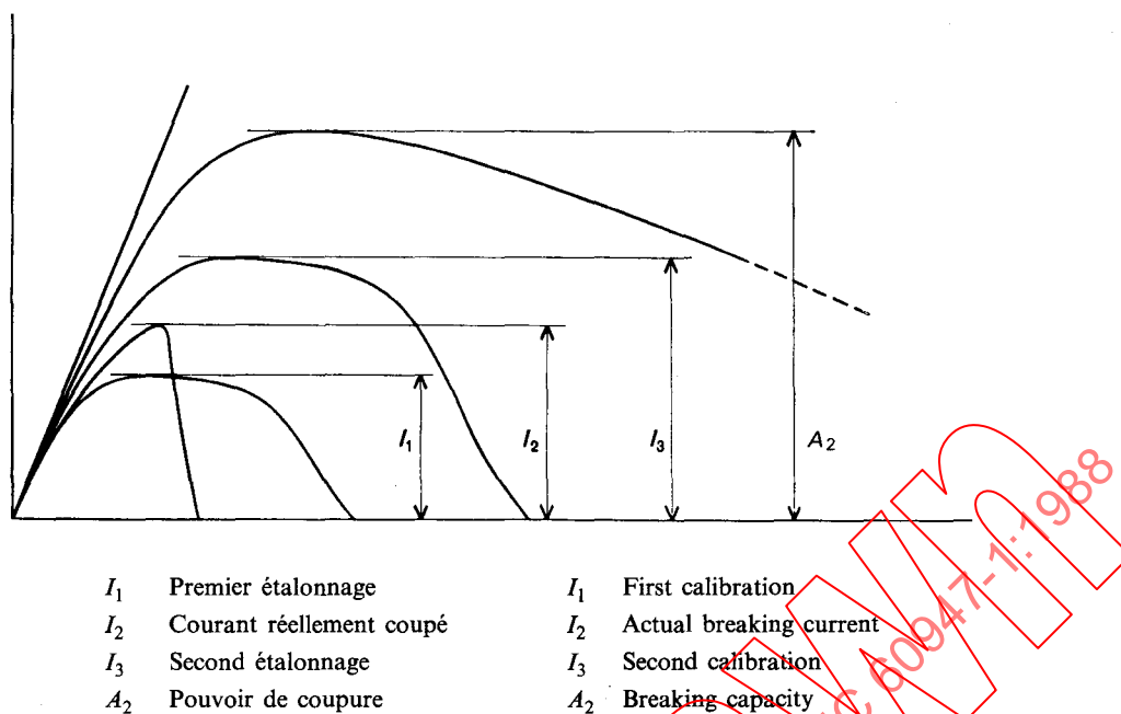
FIG. 15. — Détermination du courant coupé présumé dans le cas où le premier étalonnage du circuit d'essai a été effectué à un courant inférieur au pouvoir assigné de coupure (paragraphe 8.3.4.1.8 b)).
