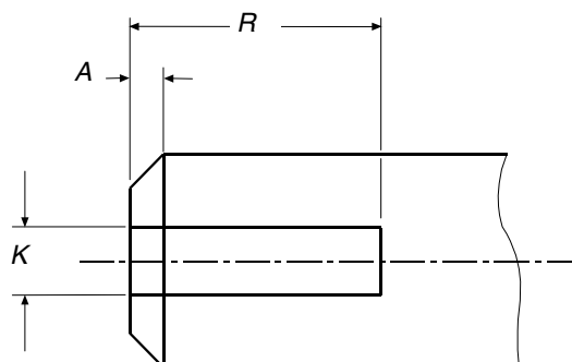
Figure E.12 – Dimensions des languettes
