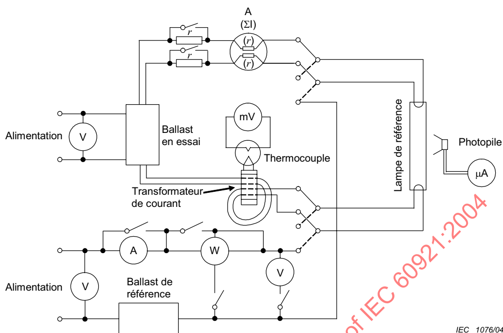
Figure A.7 – Mesure de la puissance et du courant fournis aux lampes (lampes sans starter)
