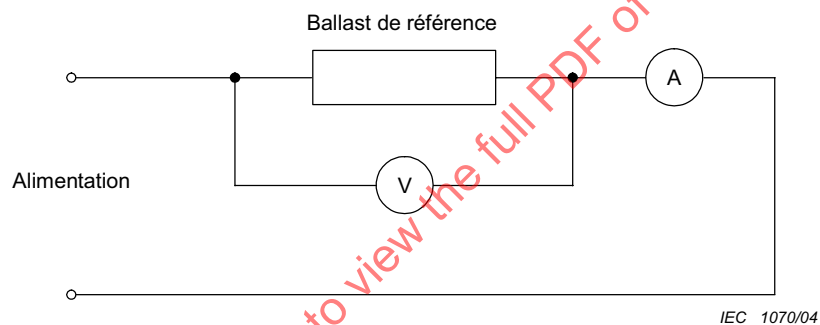
Figure A.1 – Circuit d'essai pour la mesure du rapport tension/courant
