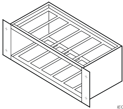
Figure 7 – Bac à cartes
