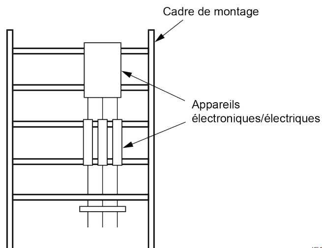
Figure 14 – Cadre de montage
