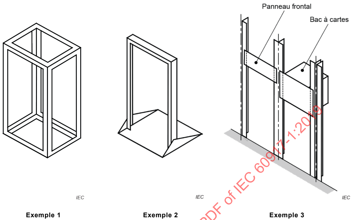
Figure 3 – Bâti
