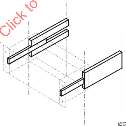
Figure 13 – Glissières télescopiques
