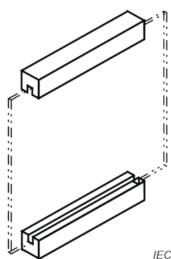
Figure 11 – Guide du bloc enfichable
