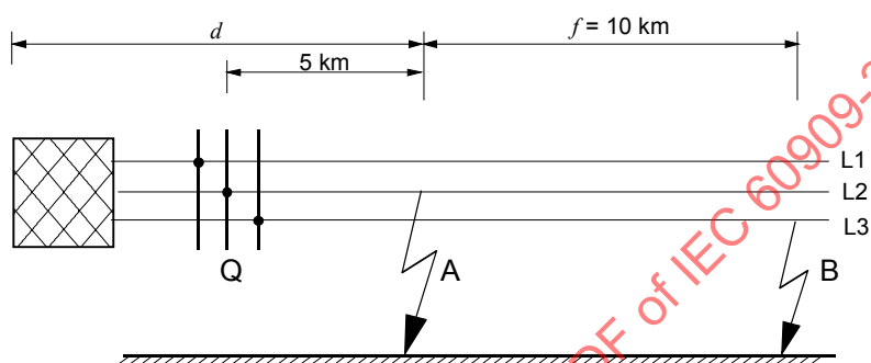
Figure A.1 – Deux courts-circuits monophasés simultanés séparés à la terre sur une seule ligne aérienne alimentée (voir Tableau 1)
