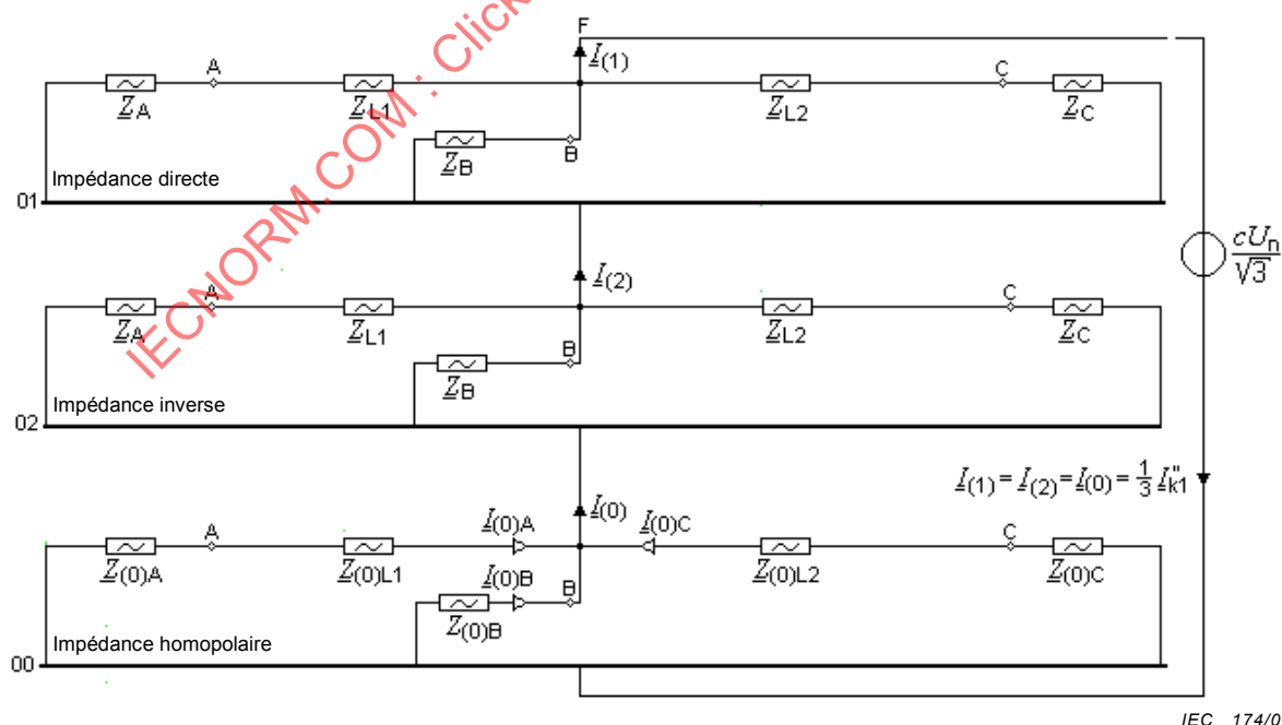
Figure B.2 – Court-circuit monphasé à la terre dans le poste B – Systèmes directs, inverses et homopolaires avec les connexions à l'emplacement F du court-circuit à l'intérieur du poste B
