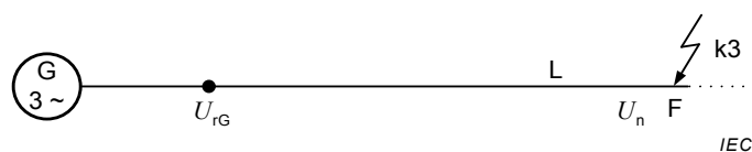
Figure 8b – Court-circuit alimenté depuis un alternateur
