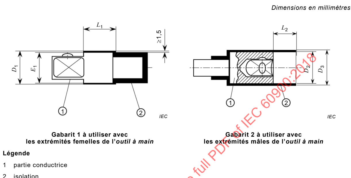
Figure 18 – Description des gabarits pour les essais diélectriques des outils à main pouvant être assemblés avec des carrés conducteurs
