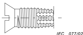
Figure 2 – Vis autotaraudeuse par enlèvement de matière (3.3.23)
