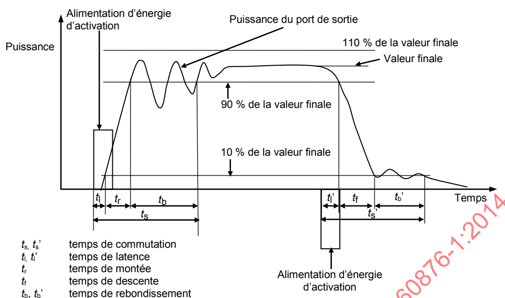
Figure 1c – Commutateur à verrouillage
