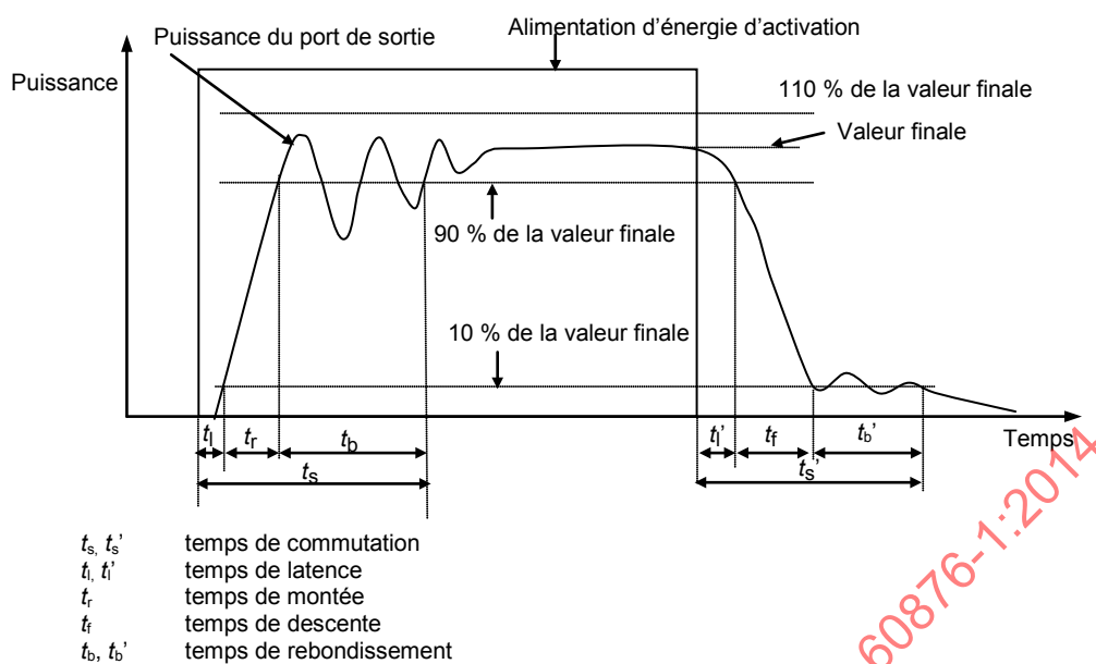
Figure 1a – Commutateur sans verrouillage, isolé par défaut
