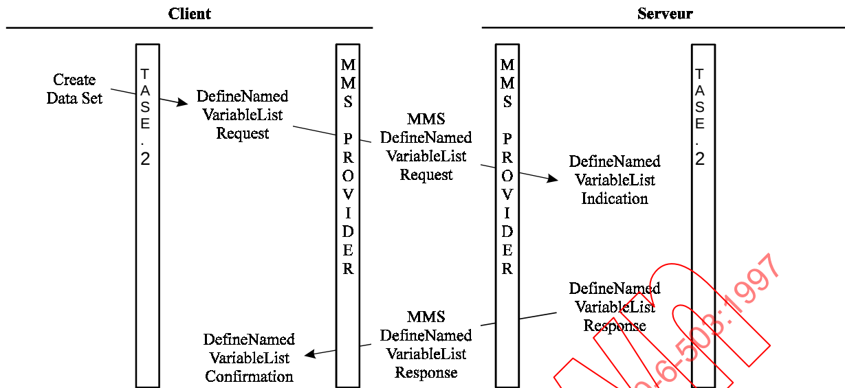
Figure 12 – Séquence de Create Data Set
