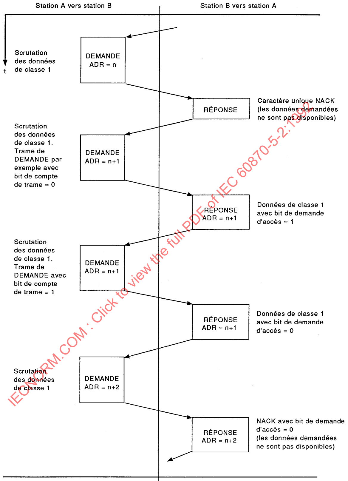
Figure 6 – Procédures de transmission non équilibrées, procédures DEMANDE/RÉPONSE non perturbées
