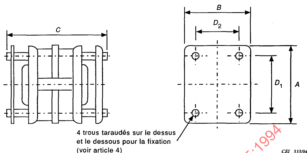
Figure 1 – Formes d'assemblage H et J pour la série Q de noyaux C
