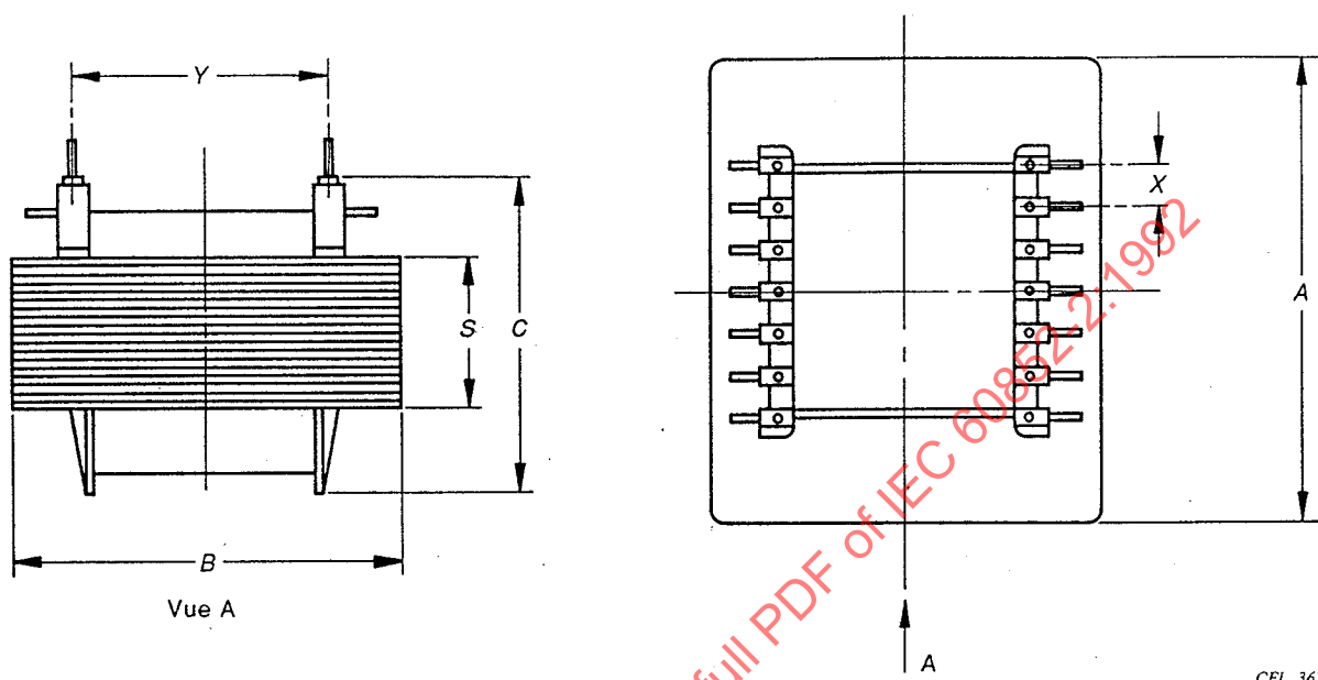
Figure 1 – Modèle de montage sur circuits imprimés de tôles découpées YEx 2-2 à YEx 2-12: configuration normale
