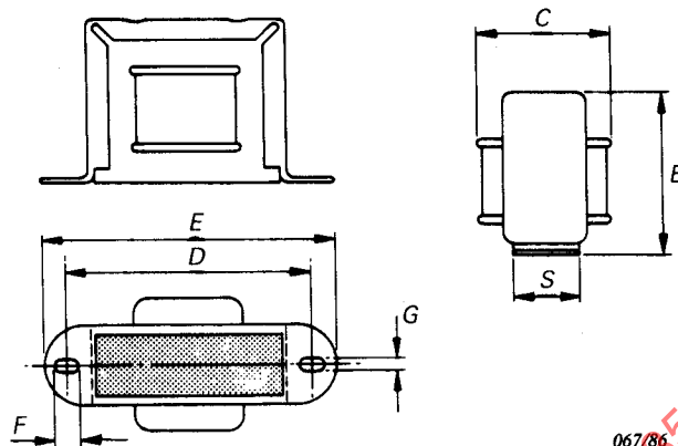
FIG. 2.— Modèle de montage à étrier pour les tôles découpées YEI 1-10 à YEI 1-25.
