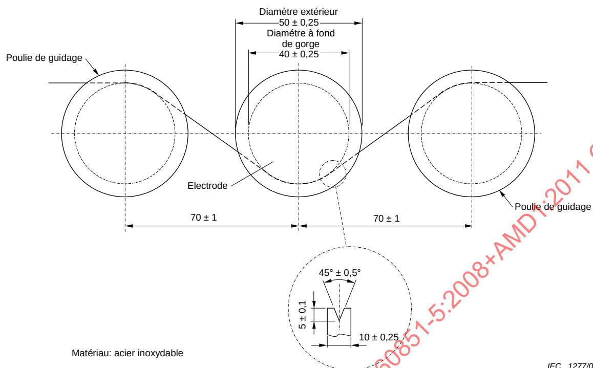
Figure 7 – Dimensions des poulies à gorge et écartement pour diamètres de fil 0,250 mm à 1,600 mm
