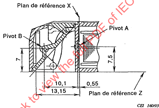
Figure 9 – Dimensions maximales du couvercle (vue latérale)
