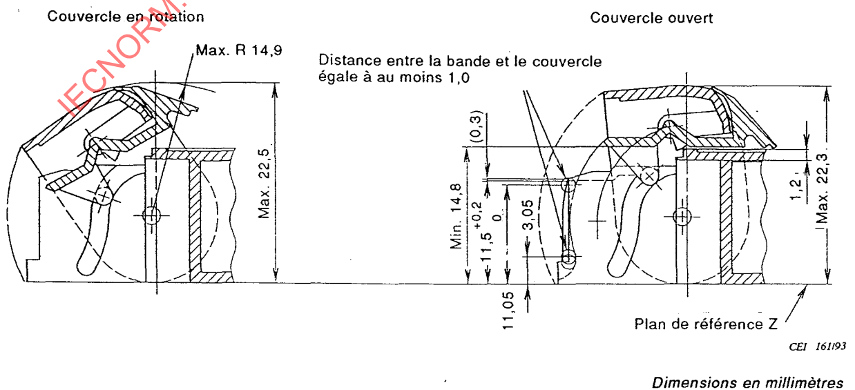
Figure 11 – Configuration du couvercle en rotation et en position ouverte
