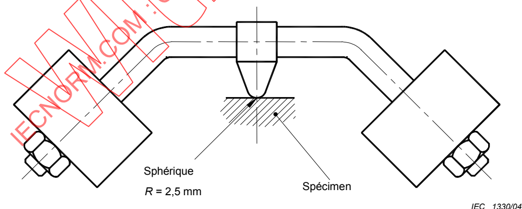
Figure 1 – Appareil pour l'essai à la bille
