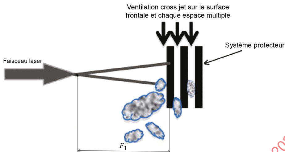
Figure D.2 – Schéma simplifié de la ventilation pour le protecteur en essai
