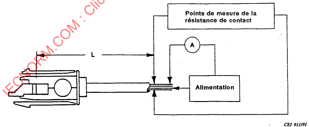
Figure 12 - Points de mesure de la résistance de contact connecteurs non accouplés
