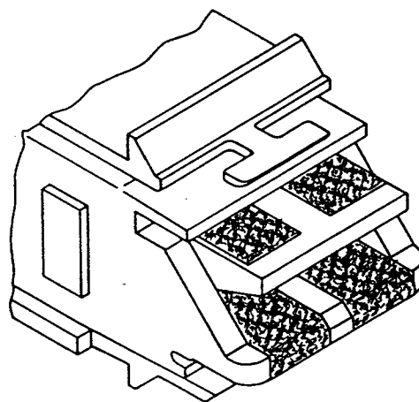
Figure 2 - Vue isométrique de la fiche
