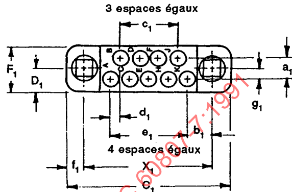
Arrangements avec 9 contacts
