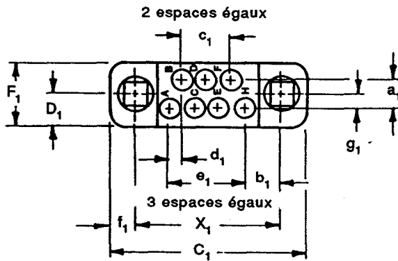
Arrangements avec 7 contacts
