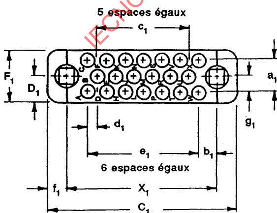
Arrangements avec 20 contacts
