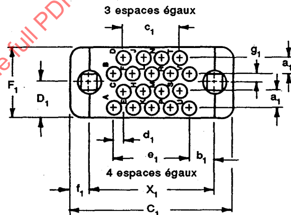
Arrangements avec 18 contacts
