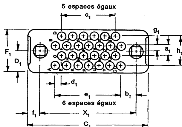
Arrangements avec 26 contacts
