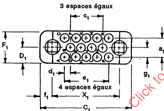
Arrangements avec 14 contacts
