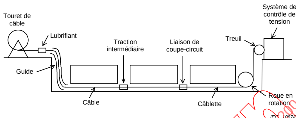
Figure A.2 – Pose de câbles à fibres optiques dans une conduite souterraine
