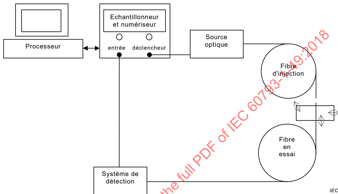
Figure 1 – Exemple d'appareillage
