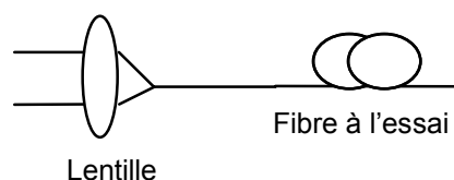
Figure A.5 – Système à lentille
