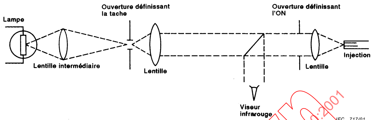
Figure A.4 – Montage optique d'injection à limitation spatiale
