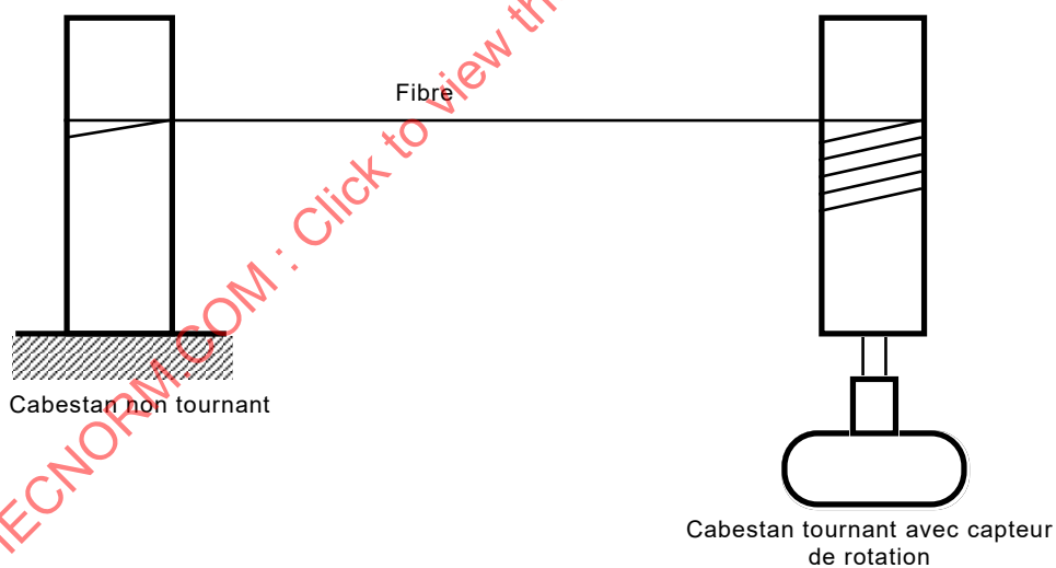
Figure A.1 – Schéma de l'appareil d'essai pour translation
