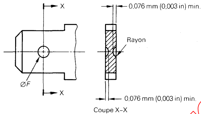
FIG. 2a. — Dimensions de l'empreinte sphérique du dispositif de verrouillage (voir figure 1, page 10).
