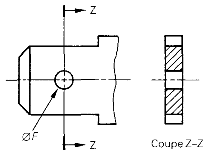
FIG. 3. — Dimensions du trou du dispositif de verrouillage (voir figure 1, page 10).
