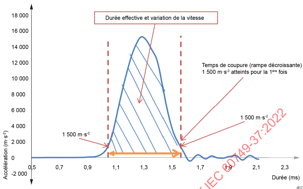
Figure 2 – Calcul de la variation de la vitesse
