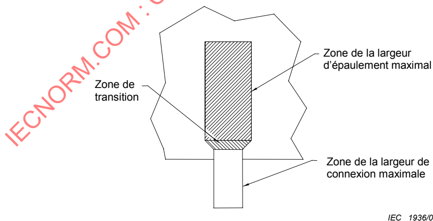
Figure 5 – Contour de la connexion J
