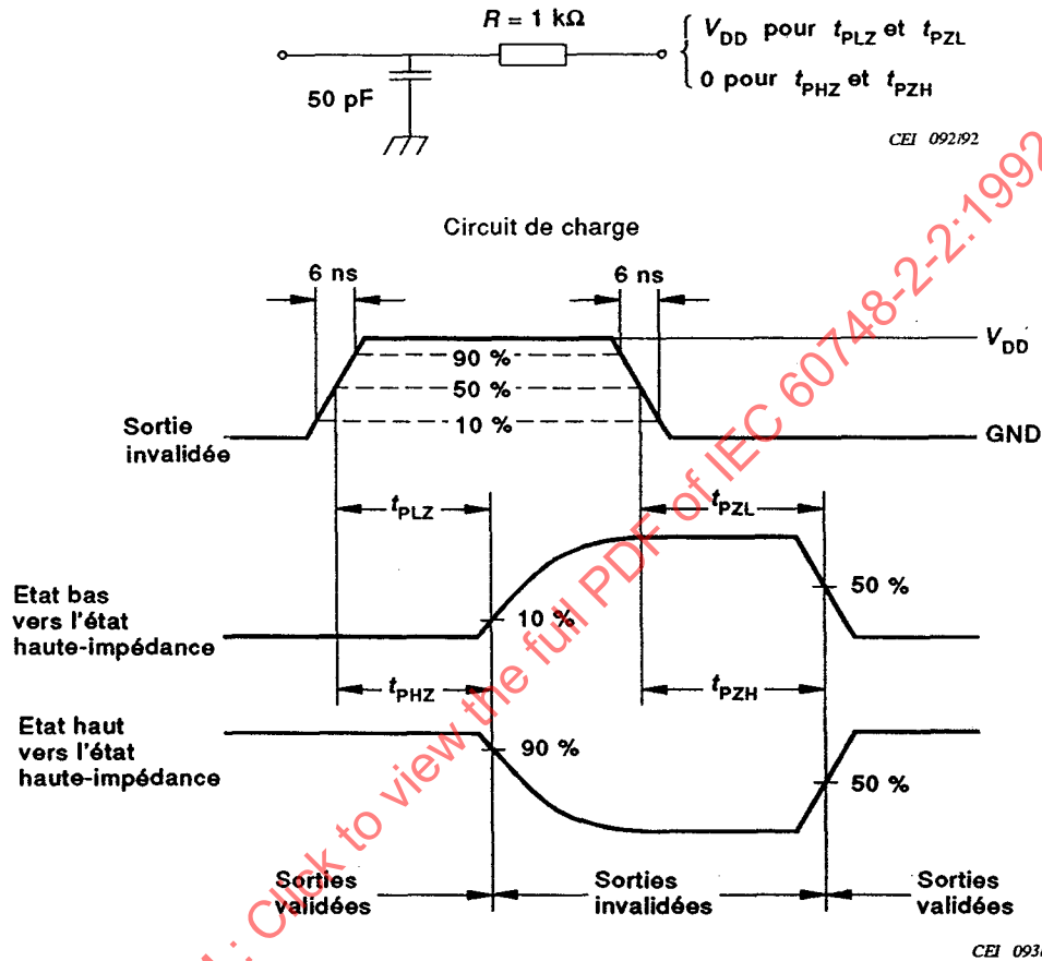
Forme d'ondes du retard de propagation pour les sorties trois états
