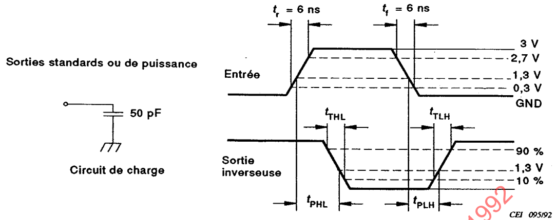
Temps de transition et temps de retard de propagation
