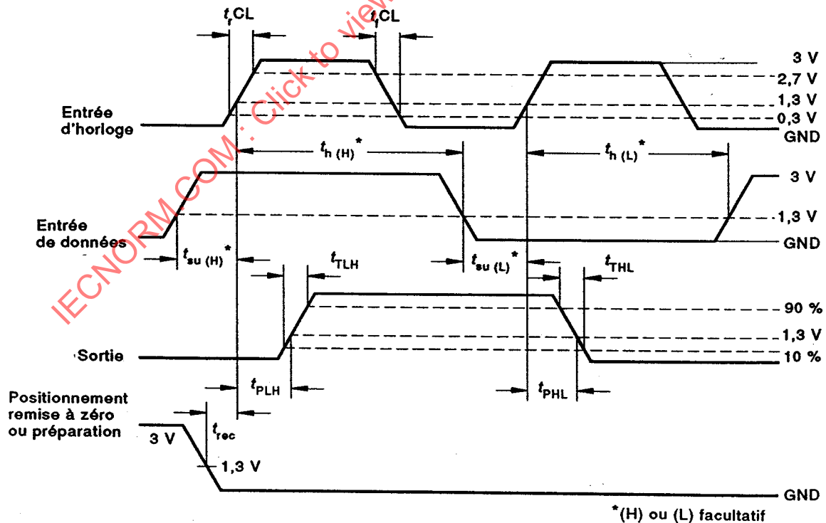
Temps de montée et de descente de l'impulsion d'horloge et largeur de cette impulsion
