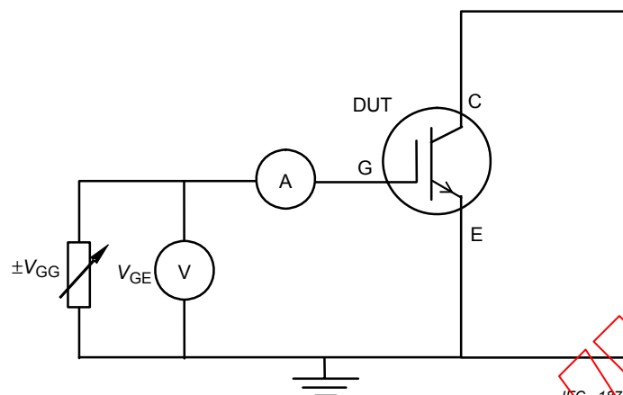
Figure 16 – Circuit pour la mesure du courant de fuite de grille
