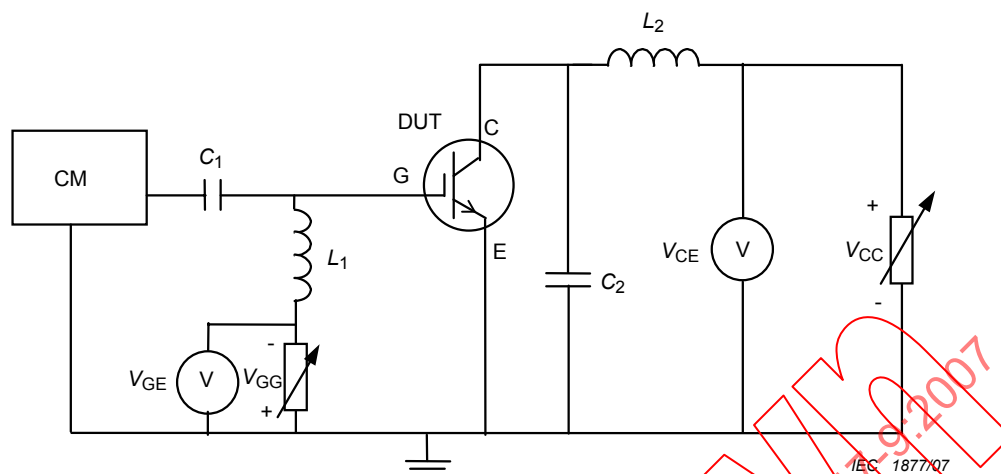
Figure 17 – Circuit de mesure de la capacité d'entrée
