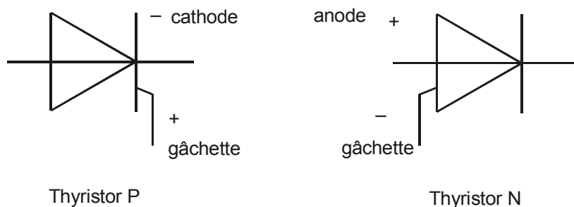
Figure 17 – Application des tensions de gâchette pour les thyristors
