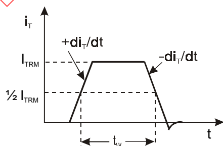
Figure 23a – Energie totale dissipée E_p pour une seule impulsion de courant à l'état passant trapézoïdale de durée t_w et d'amplitude I_{TRM}
