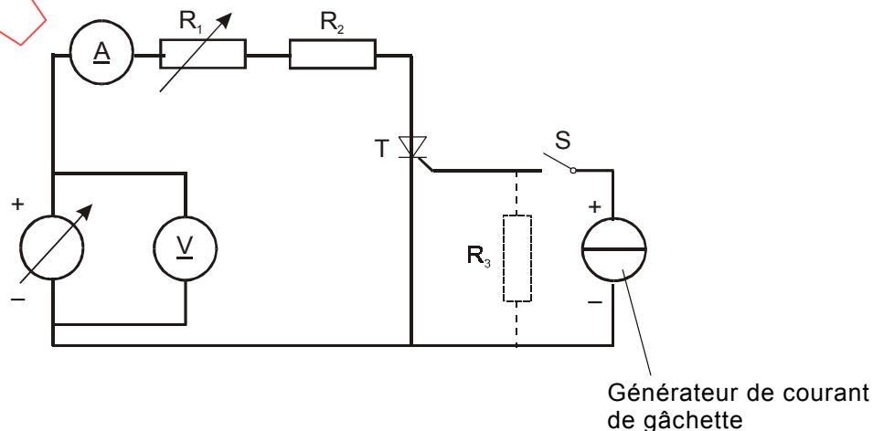
Figure 32 – Circuit de mesure du courant de maintien
