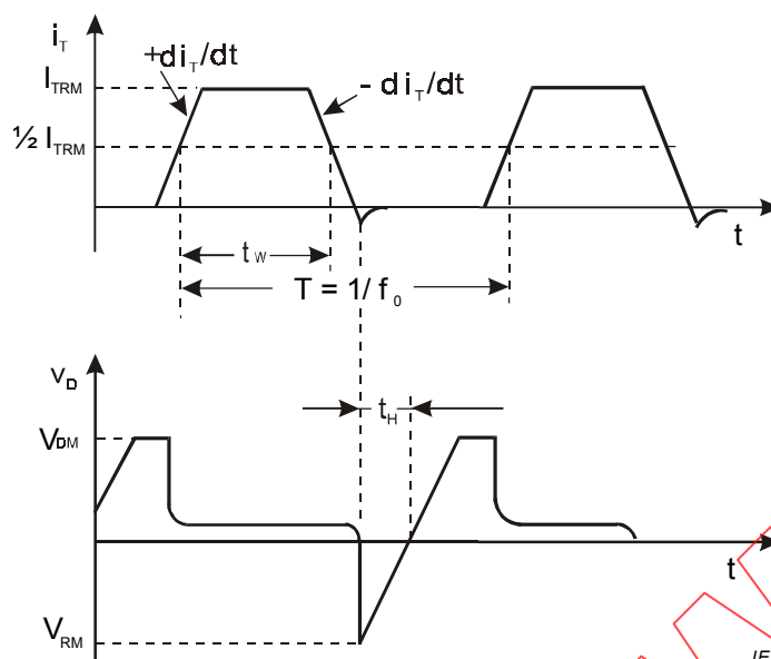
Figure 19c – Formes d'onde typiques du courant et de la tension pour impulsions de courant à l'état passant trapézoïdales; t_H est l'intervalle de suppression (voir 3.9.14)
