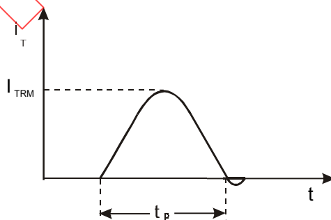
Figure 22a – Energie totale dissipée E_p pour une seule onde demi-sinusoïdale de l'impulsion de courant à l'état passant de durée t_p et d'amplitude I_{TRM}
