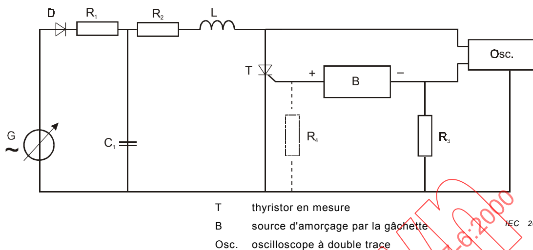
Figure 37 – Circuit de mesure du retard à la croissance commandée par la gâchette et du temps d'amorçage par la gâchette
