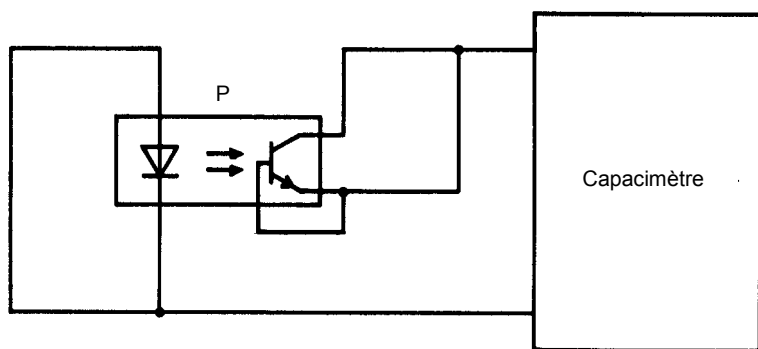
Figure 4 – Circuit de mesure pour capacité entrée-sortie
