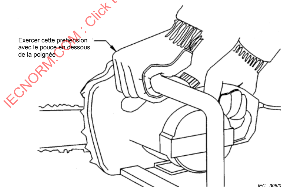
Figure 103 – Préhension de la scie à chaîne
