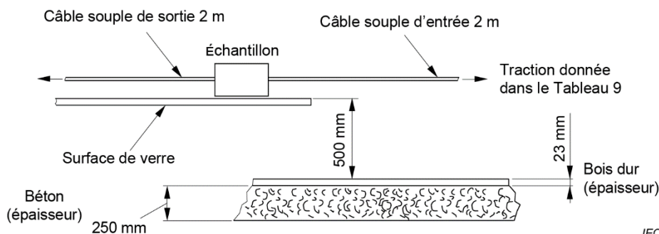
Figure 7 – Essai de chute pour dispositifs de commande séparés
