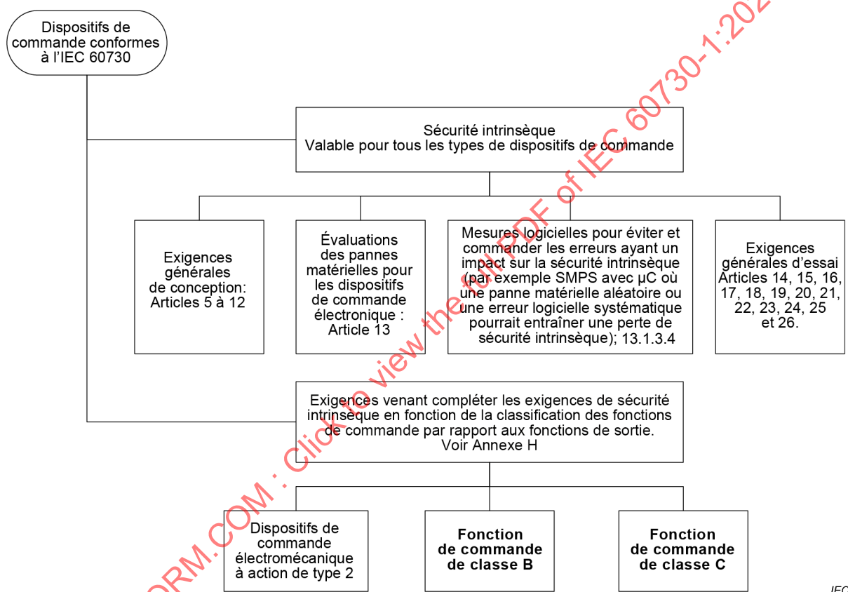
Figure 2 – Structure du document concernant la sécurité intrinsèque et la sécurité fonctionnelle
