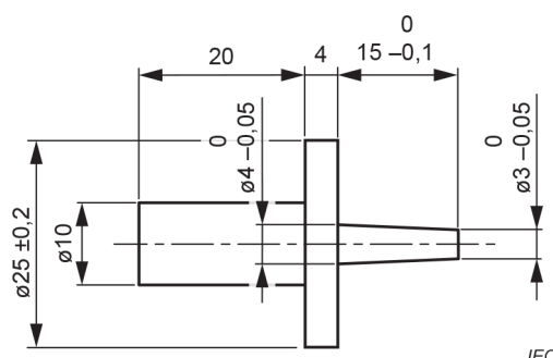
Figure 4 – Broche d'épreuve de calibre 13 de l'IEC 61032:1997
