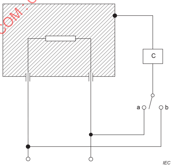
Figure 19 – Schéma pour la mesure du courant de contact à la température de fonctionnement pour connexion monophasée des dispositifs de commande de la classe II
