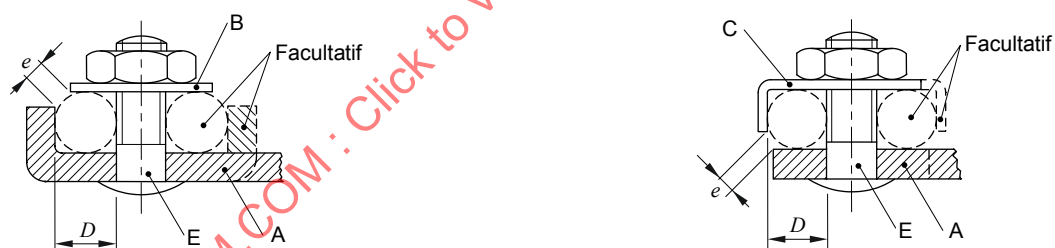
Bornes à goujon fileté
