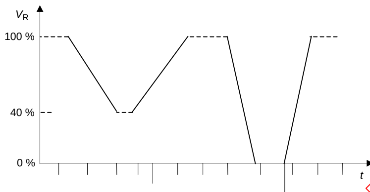
Figure H.26.5.4.2 – Essai de variation de tension
