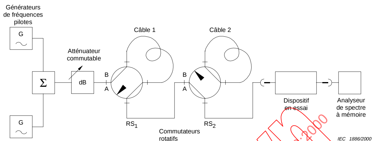
Figure 6 – Mesure de la réponse à une variation instantanée du dispositif de commande automatique de gain
