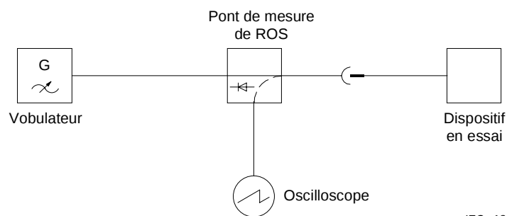
Figure 1 – Mesure du facteur d'adaptation
