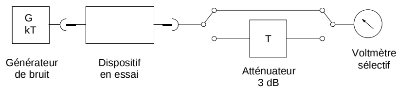
Figure 8 – Mesure du facteur de bruit
